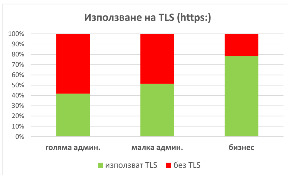
Фигура 7. Използване на защитена връзка https: (TLS)
